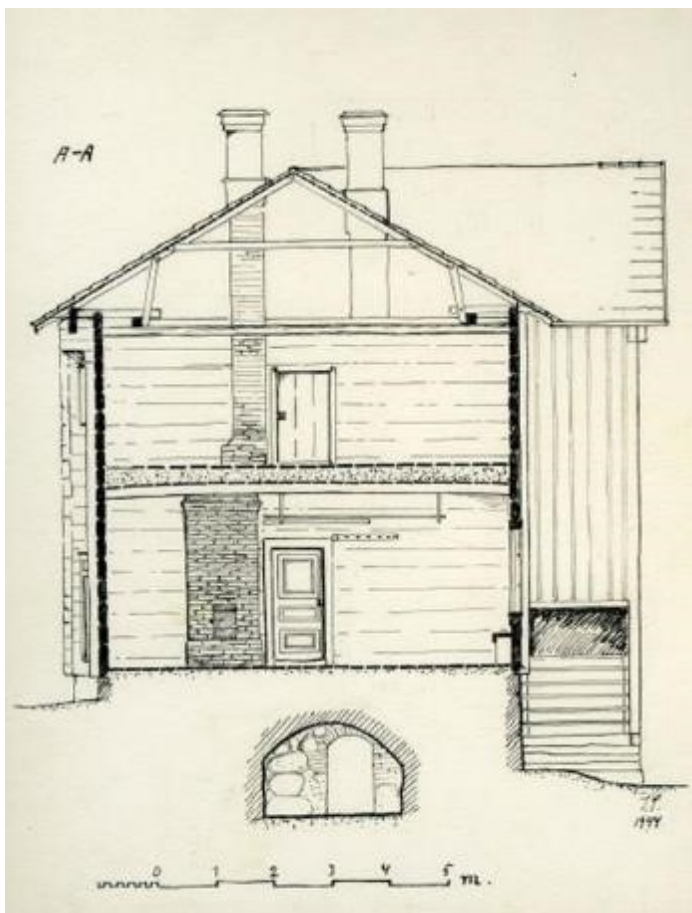
Irja Sahlbergin piirros vanhan päärakennuksen poikkileikkauksesta, jossa näkyy myös rakennusta vanhempi kellari. Kuva: Turun museokeskus / Finna.
