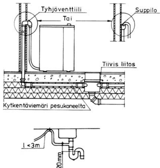
Kuva 7. Esimerkkejä kotitalouskäyttöön tarkoitettujen pesu- tai astianpesukoneen viemärintavoista.
