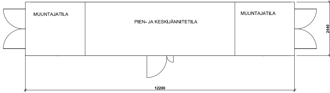
POHJA
