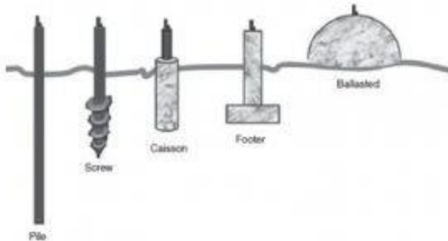
Kuva 18: Aurinkovoimalan maatelineen perustamisvaihtoehdot [12].
