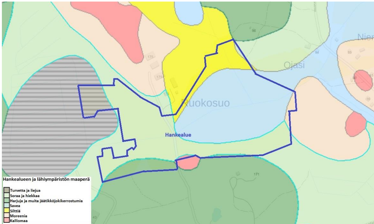
Kuva 6: Hankealueen (sininen rajaus) ja lähialueiden maaperärakenne [4].
