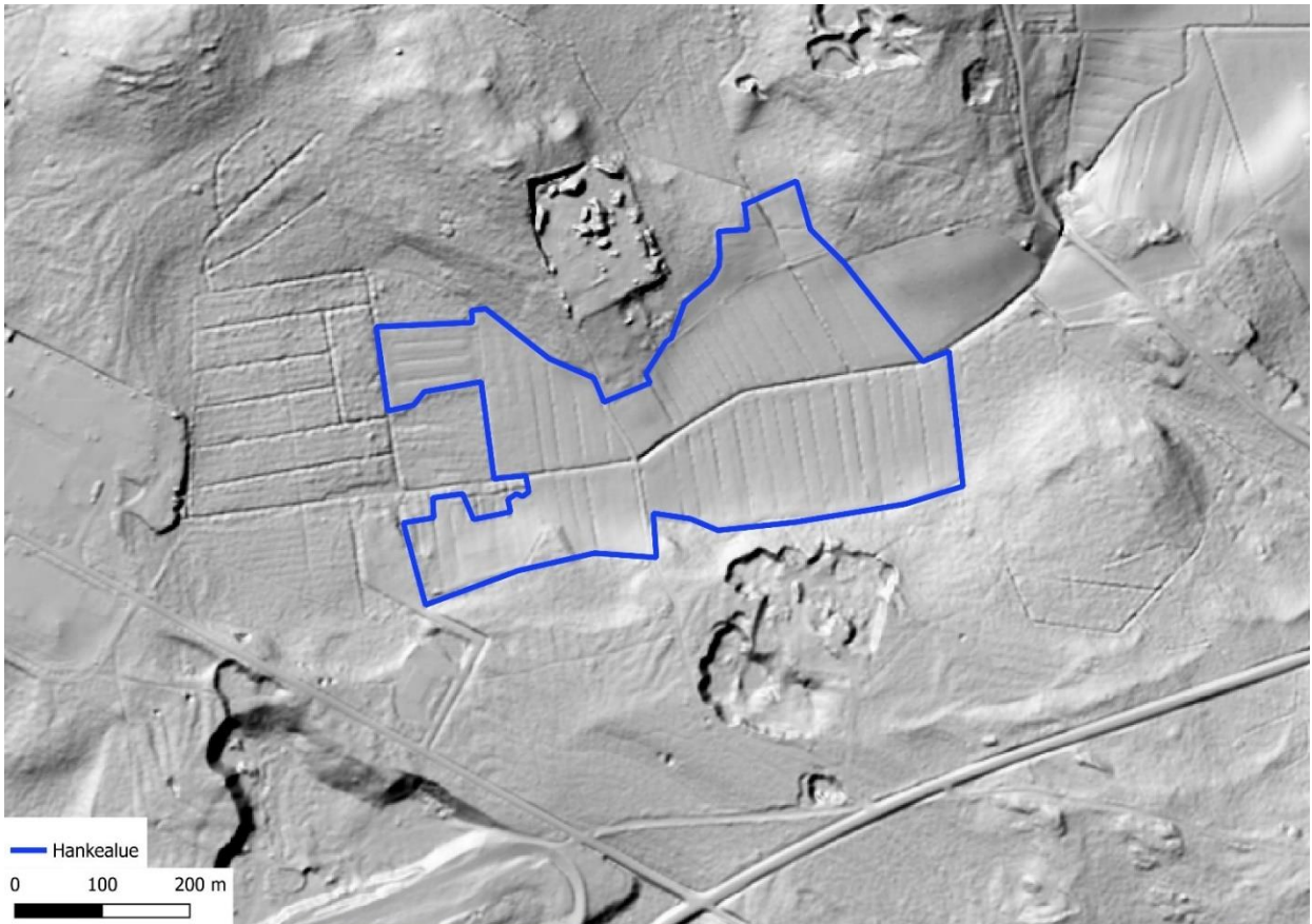
Kuva 8: Maastonmuodot hankealueella [4].
