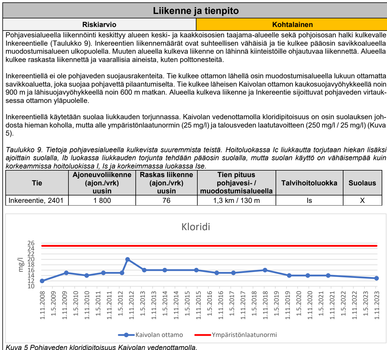
Kuva 5 Pohjaveden kloridipitoisuus Kaivolän vedenottamolla.
